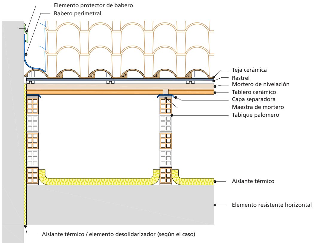
SECCIÓN TRANSVERSAL
