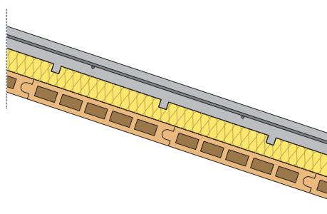
Figura 6.46 Colocación de losa sobre el aislamiento ranurado
