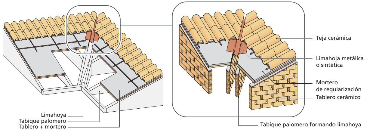
Figura 6.54. Limahoya
